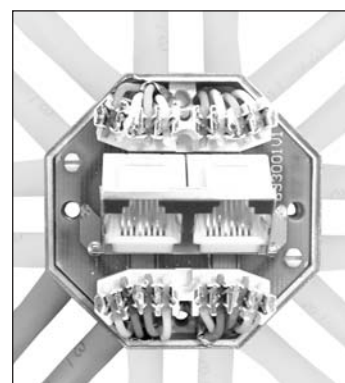
Kabelzuführung von 8 Seiten.
